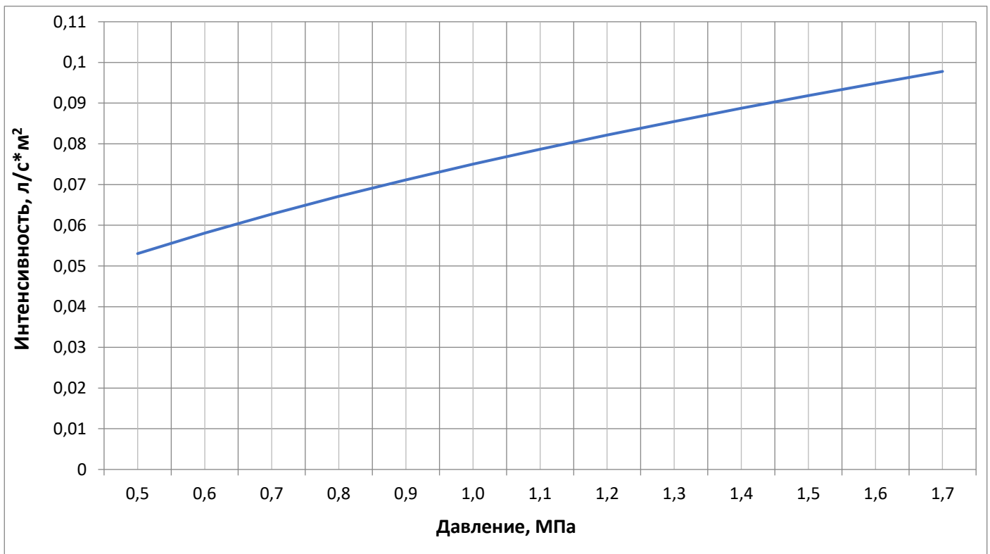
График зависимости интенсивности орошения от давления на площади 12 м 2 , защищаемой одним оросителем с высоты 2,5 м
